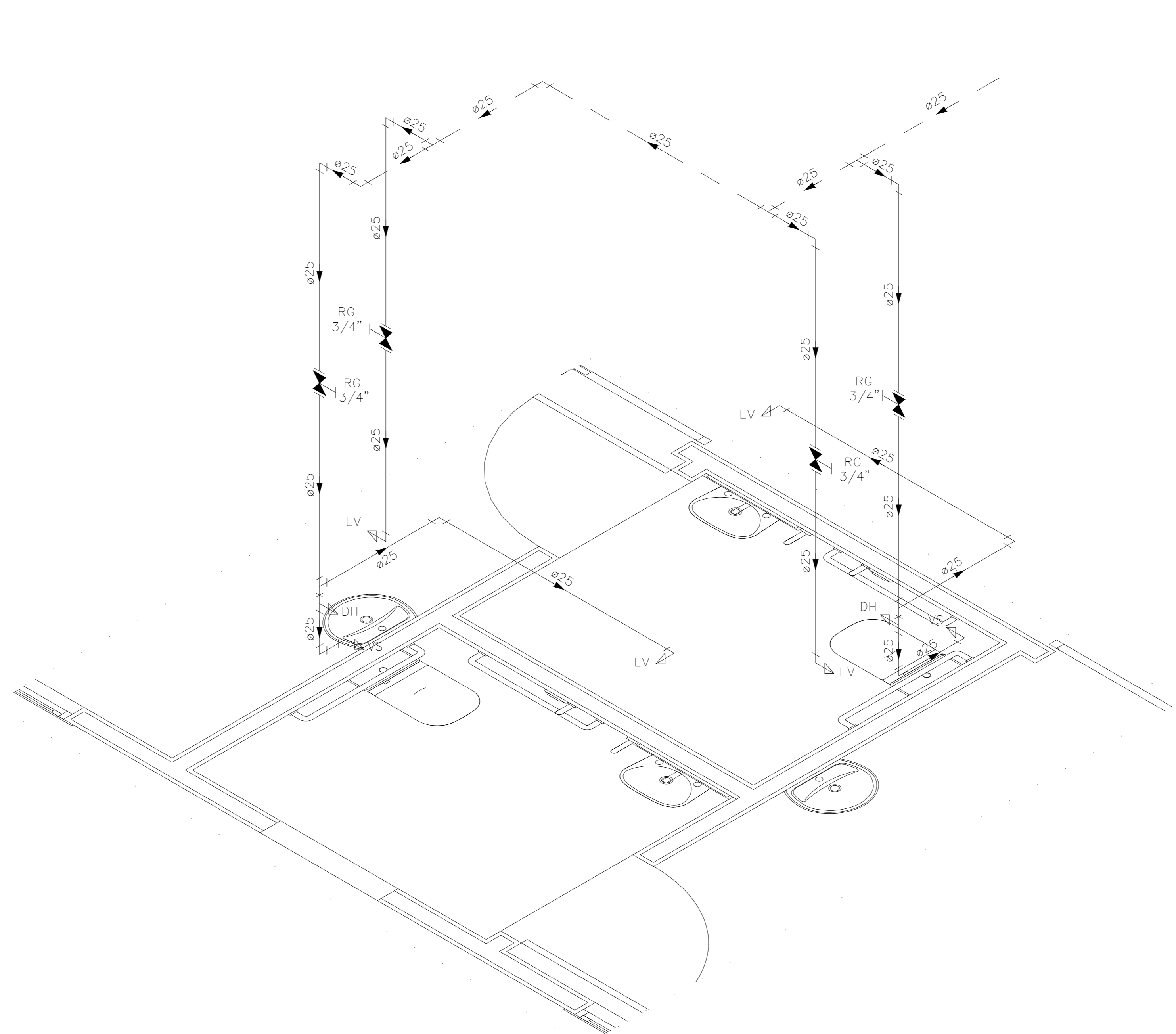
DETALHE HID-23 ESCALA 1:25
