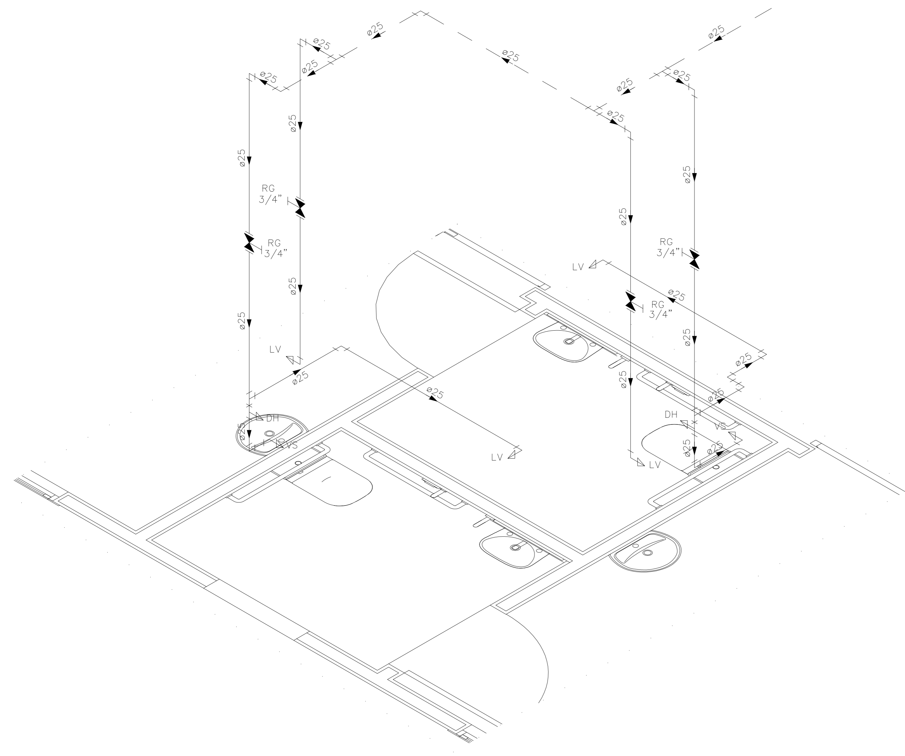
DETALHE HID-22 ESCALA 1:25
