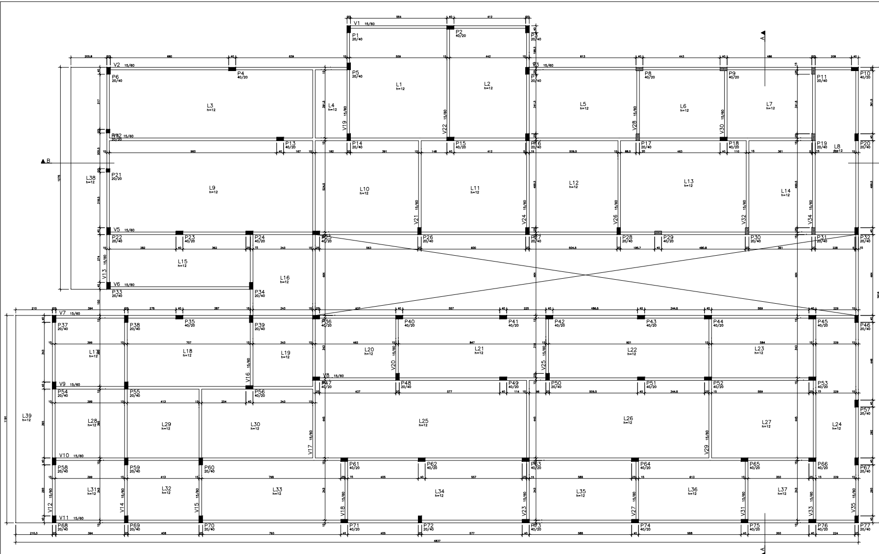
FORMAS DA COBERTURA ESCALA 1:50
