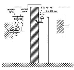
DETALHE CORRIMÃO SEM ESCALA
