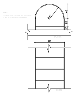
DETALHE ESCADA MARINHEIRO SEM ESCALA
