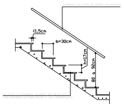
DETALHE DEGRAUS DAS ESCADAS SEM ESCALA
