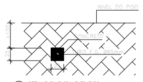
DETALHE ENVELOPAMENTO TUBO SEM ESCALA
