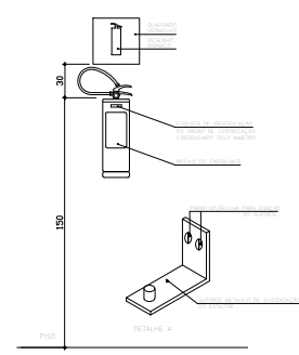
DETALHE EXTINTOR NA PAREDE SEM ESCALA
