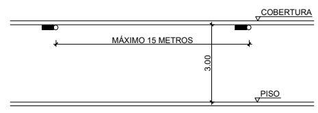
DETALHE DE INSTALAÇÃO ILUMINAÇÃO EMERGÊNCIA SEM ESCALA
