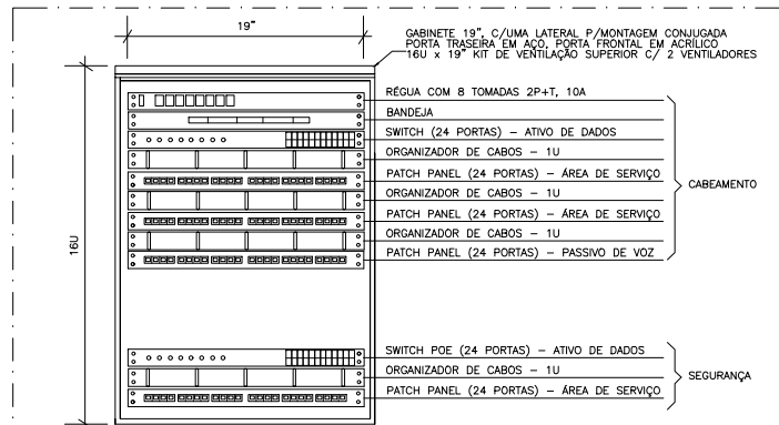
DIAGRAMA ESQUEMÁTICO DO RACK R01 E R02 SEM ESCALA
